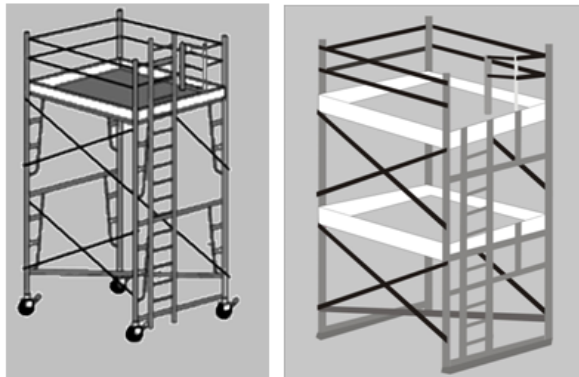
Figura 5 Andamios tipo torre o estructura
