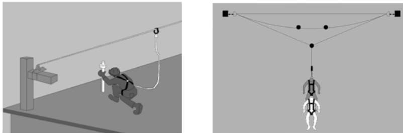
Figura 3 Líneas de vida horizontales
