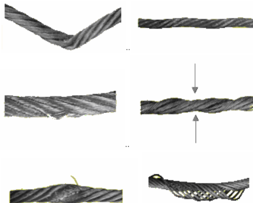
Figura 9 Ejemplos de condiciones inseguras en cables
